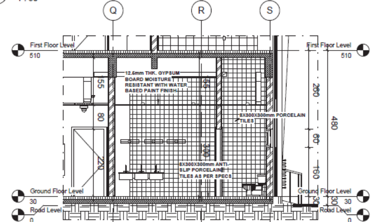
6 TOILET DETAILS SEC-GF72 1:50 AR-032
