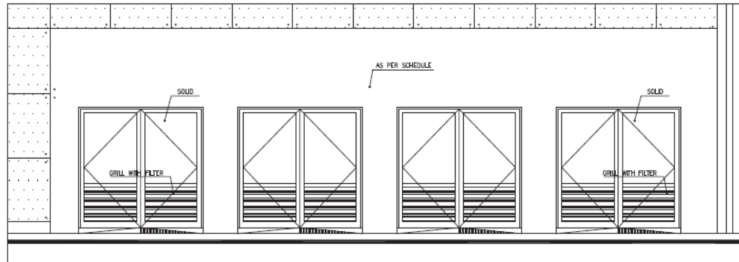
ELEVATION (1)
