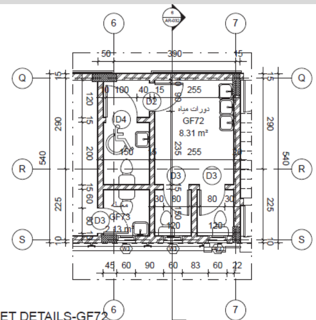
3 TOILET DETAILS-GF72 1:50 AR-032
