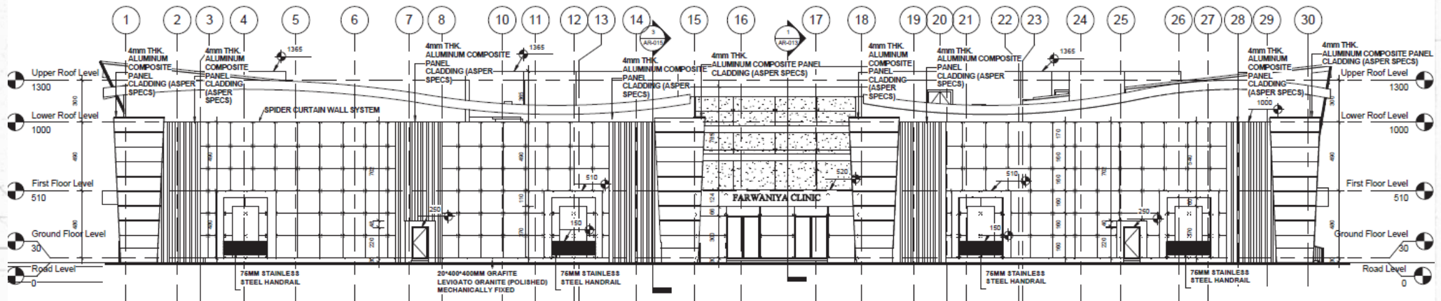
ELEVATION 1 1:150
