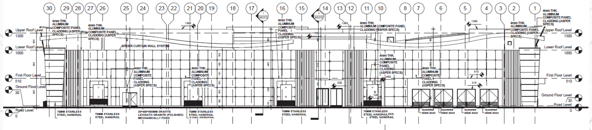
ELEVATION 3 1:150
