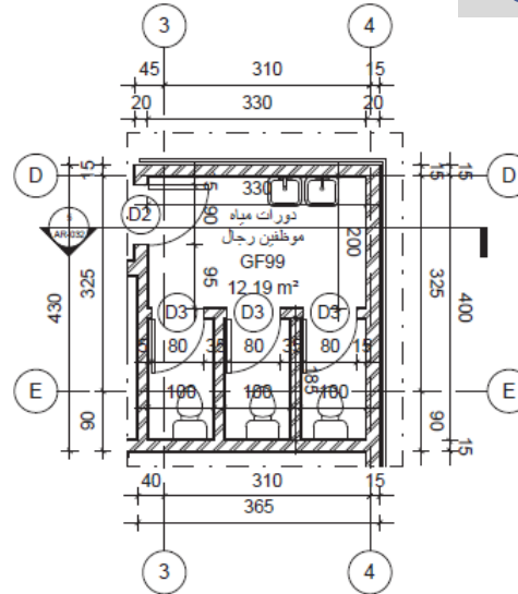
2 TOILET DETAILS-GF99 1:50 AR-032
