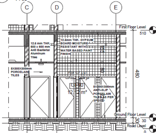
4 TOILET DETAILS SEC-GF90 1:50 AR-032
