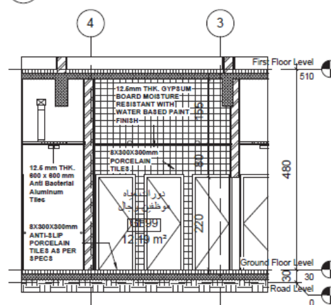
5 TOILET DETAILS SEC-GF99 1:50 AR-032
